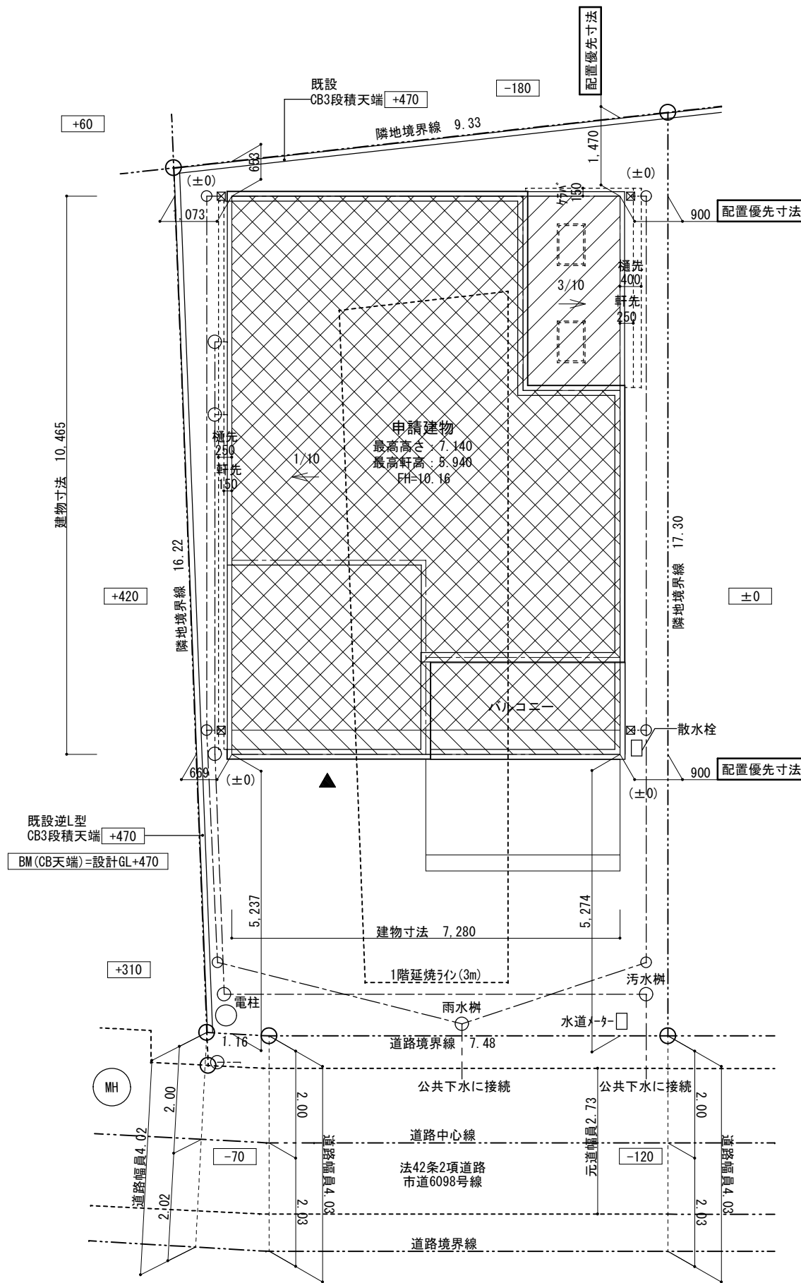
配置図 S=1/100
