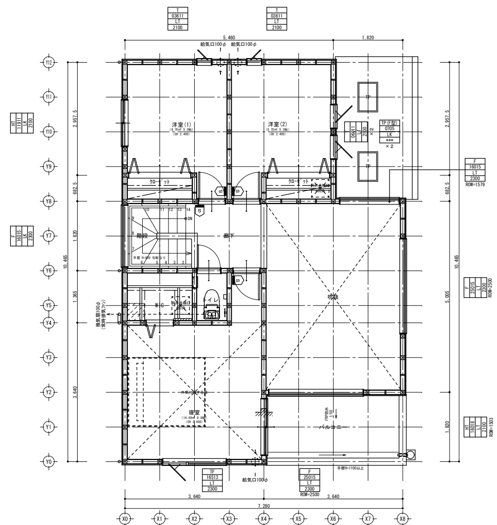
2階平面図
